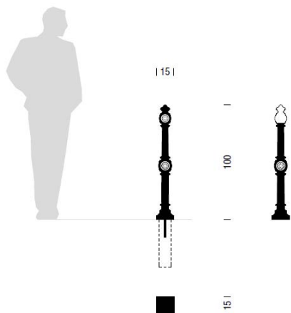
Visok stebriček tip Stara Ljubljana
