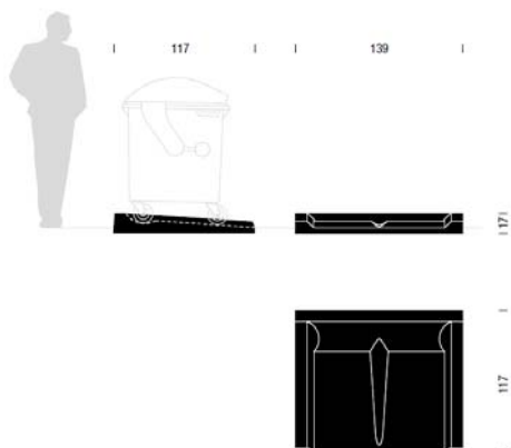
Podstavek za zabojnike
