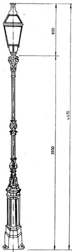
Drog tip Zvezda s svetilko tip Gornji trg
