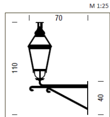
Konzolna svetilka tip Gornji trg - dolga
